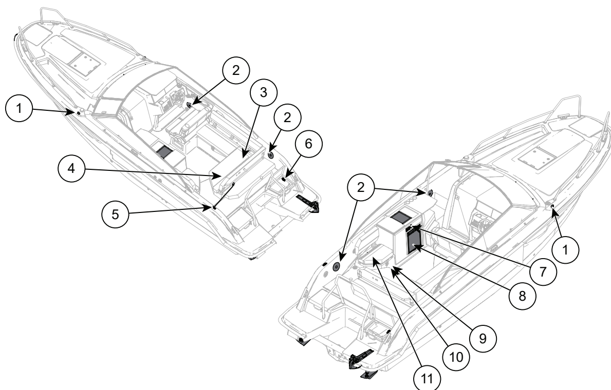
Figur 8.3 Yamarin 80 DC elektrisk utstyr
