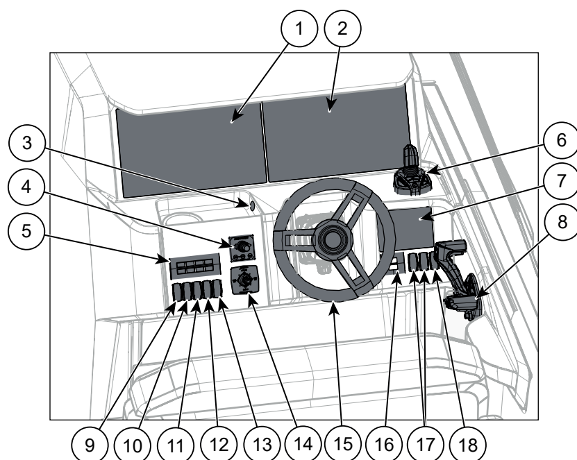
Figur 5.1 Yamarin 80 DC styrestasjonskontroller
