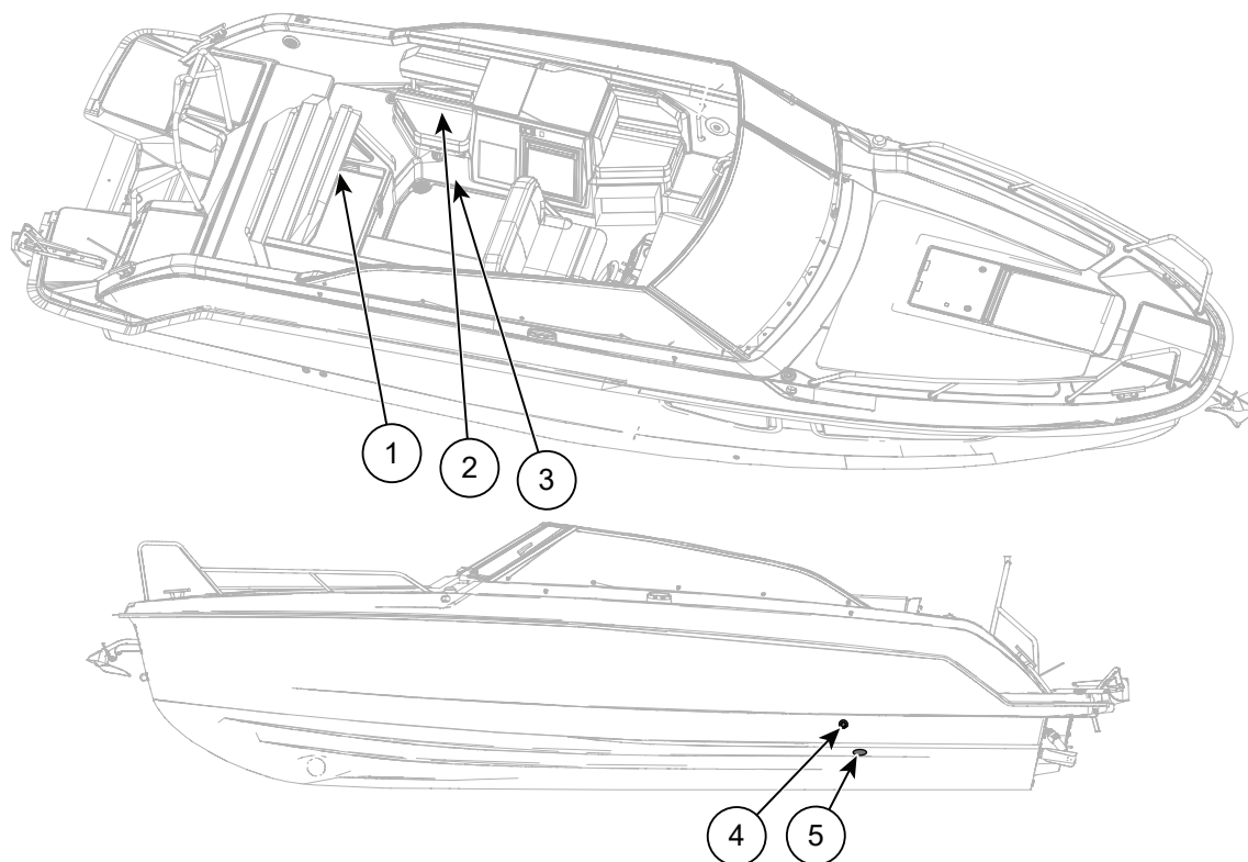
Figur 11.3 Yamarang 80 DC klimaanlegg
