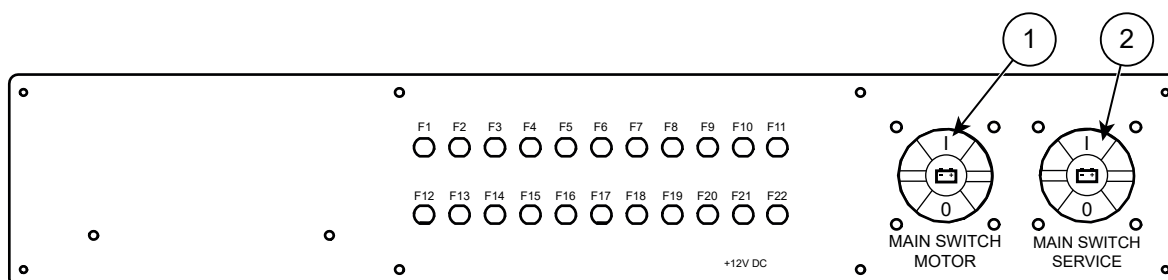
Figur 8.1 Yamarin 80 DC hovedbrytere og sikringspanel
