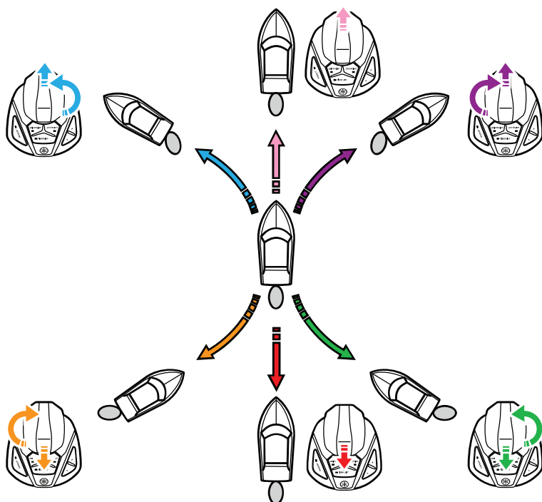
Figur 5.6 Bruk av styrespak i en båt med én motor
