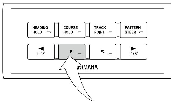
Figur 5.7 Autopilot-kontrollpanel
