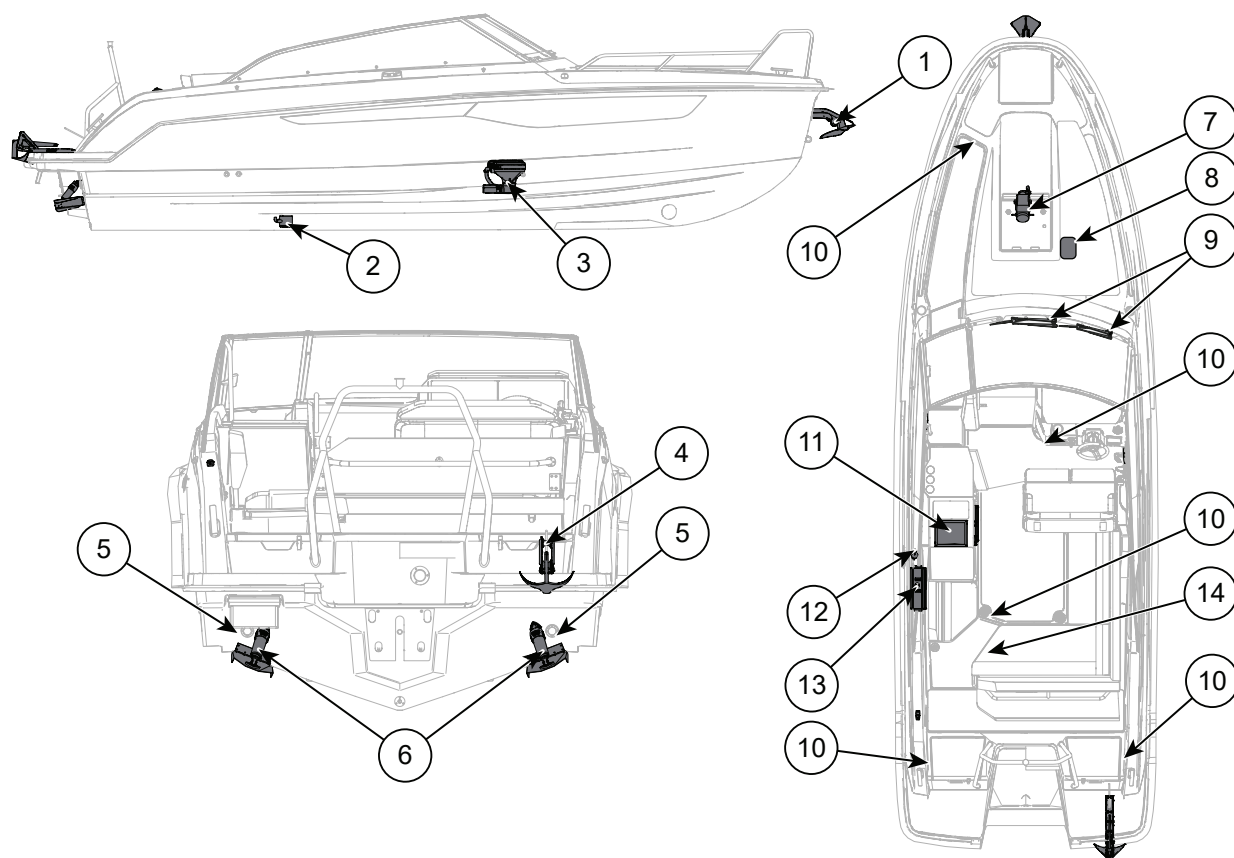
Figur 8.2 Yamarin 80 DC elektrisk utstyr
