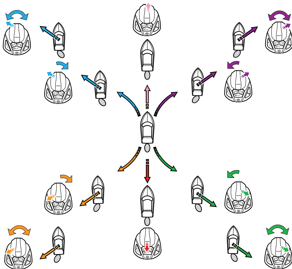
Figur 5.9 Bruk av styrespak med integrert kontroll av baugpropell
