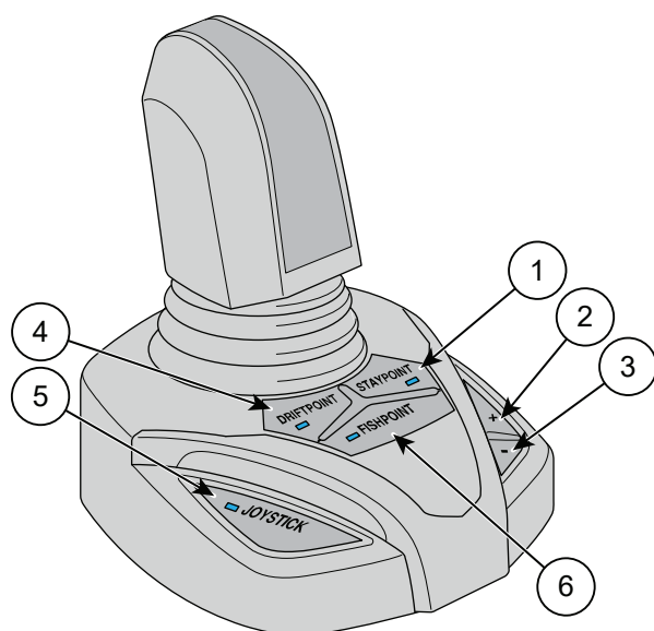
Figur 5.5 Styrespak og funksjonsknapper
