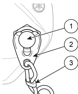
Figur 5.4 Nødbryter
