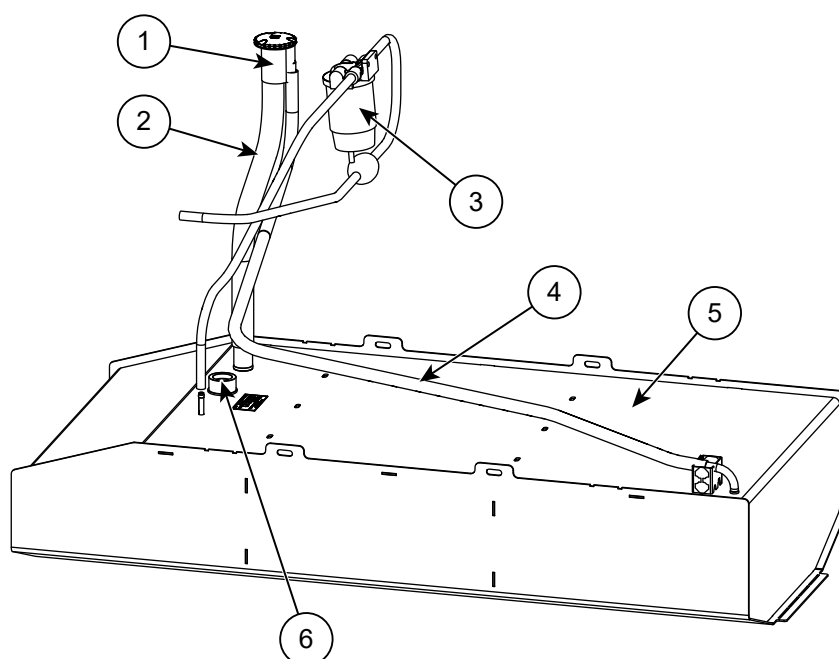
Figur 6.1 Drivstoffsystem
