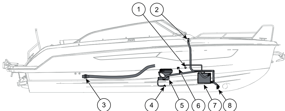
Figur 11.1 Yamarin 80 DC septiksystem
