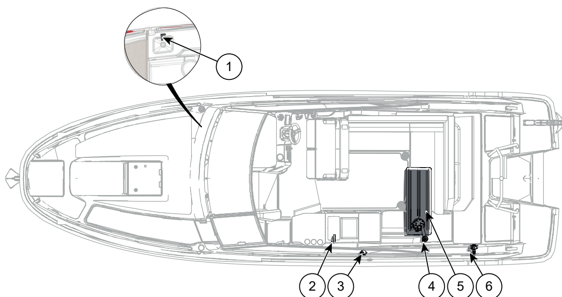
Figur 10.1 Yamarin 80 DC ferskvannssystem
